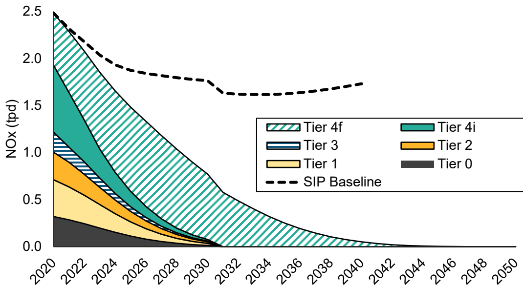
Figure 38 - Statewide CHE NOx Emissions: MSS Scenario
